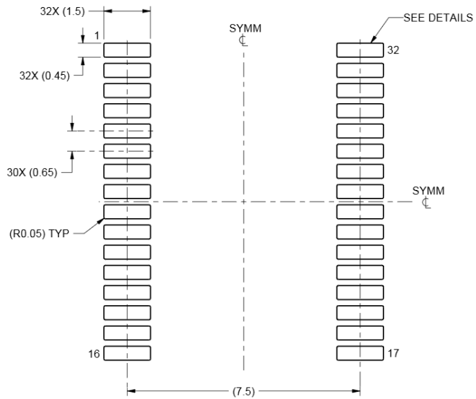
LAND PATTERN EXAMPLE SCALE: 8X
