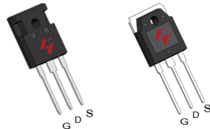
TO-247A-3L
