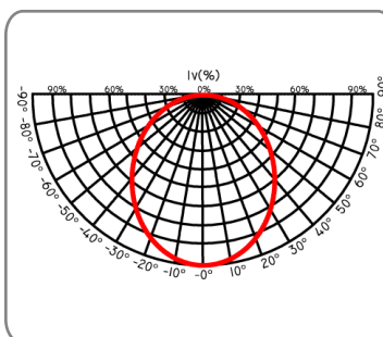
Curva de Distribucion luminosa
